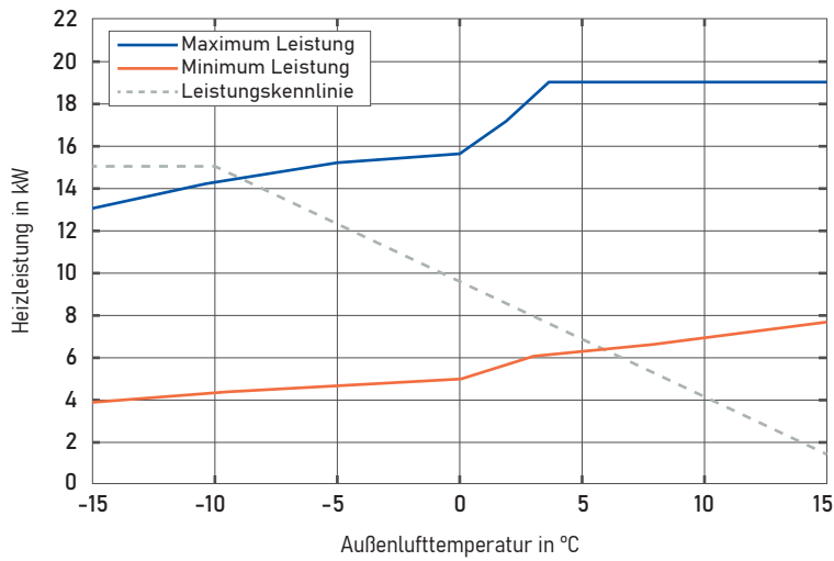
Abb. 5: Leistungsbereich der EU15L je nach Außenlufttemperatur bei 5K Spreizung und 85 % Luftfeuchte (oben: 35 °C Vorlauftemperatur / unten: 55 °C Vorlauftemperatur) mit empfohlener Leistungskennlinie nach EN 14825.
