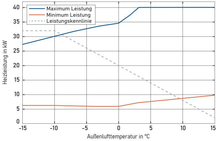
Abb. 9: Leistungsbereich der EU35L je nach Außenlufttemperatur bei 5K Spreizung und 85 % Luftfeuchte (oben: 35 °C Vorlauftemperatur / unten: 55 °C Vorlauftemperatur) mit empfohlener Leistungskennlinie nach EN 14825.
