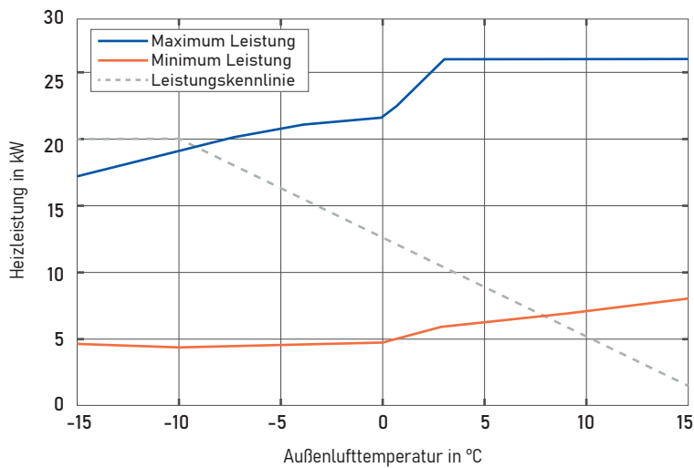
Abb. 7: Leistungsbereich der EU20L je nach Außenlufttemperatur bei 5K Spreizung und 85 % Luftfeuchte (oben: 35 °C Vorlauftemperatur / unten: 55 °C Vorlauftemperatur) mit empfohlener Leistungskennlinie nach EN 14825.
