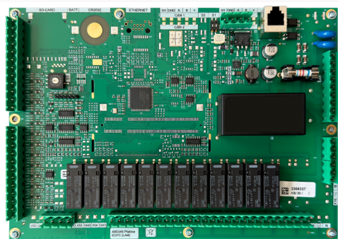
Abb. 2: AHC-Hydraulikregeleinheit
