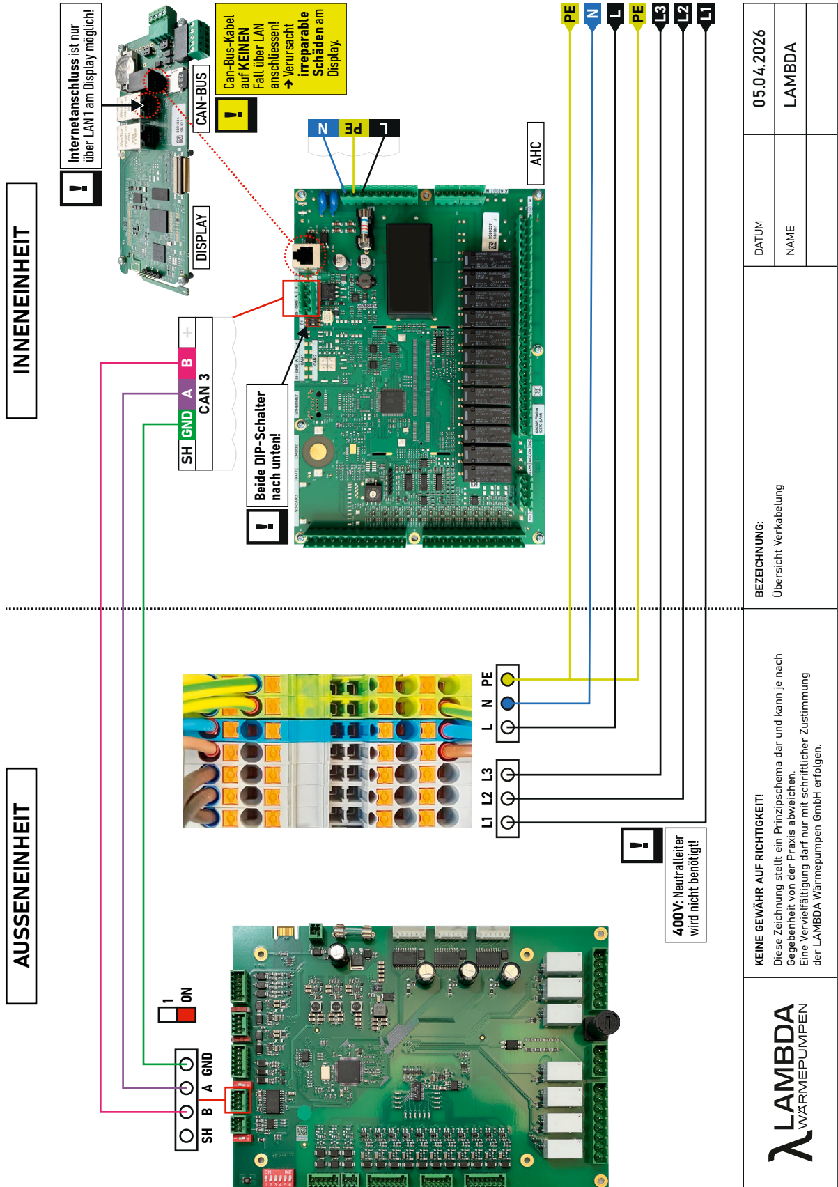
Abb. 4: Übersicht Verkabelung
